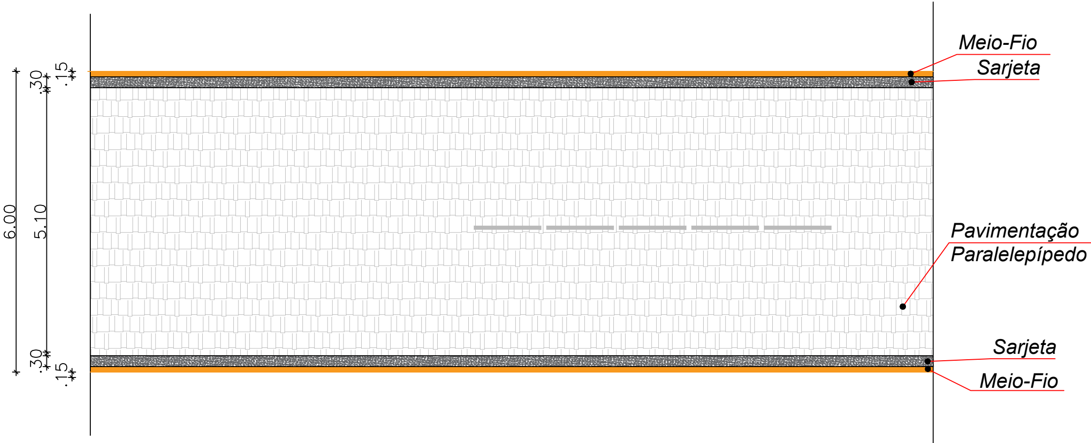
PLANTA BAIXA - TRECHOS COM LARGURA DE 6,00 M
