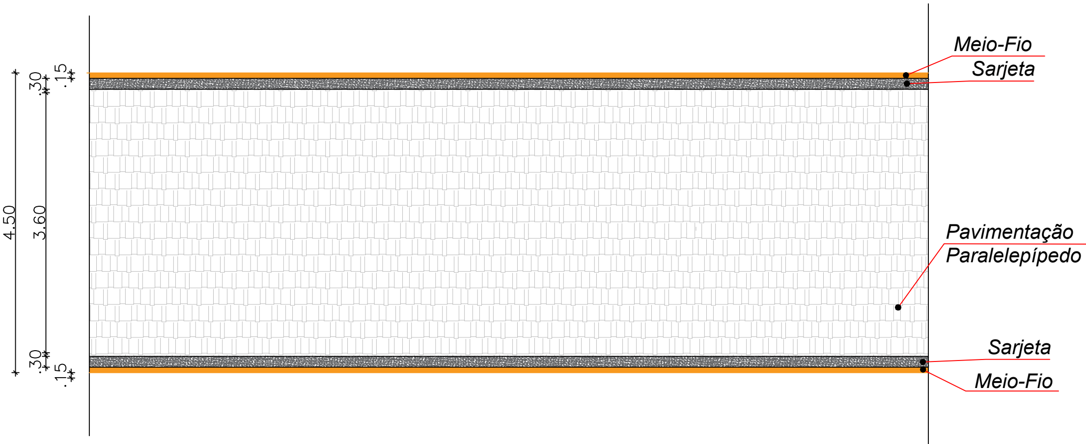
PLANTA BAIXA - TRECHOS COM LARGURA DE 4,50 M
